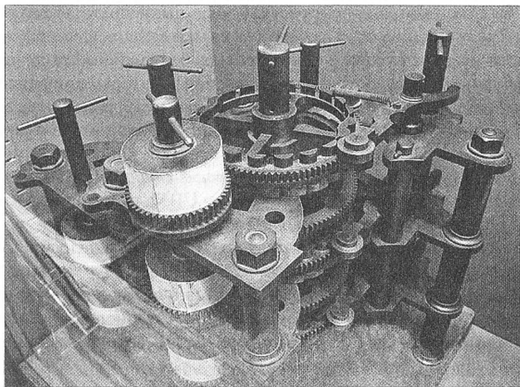
Рис. 3.1. Машина Бэббиджа
