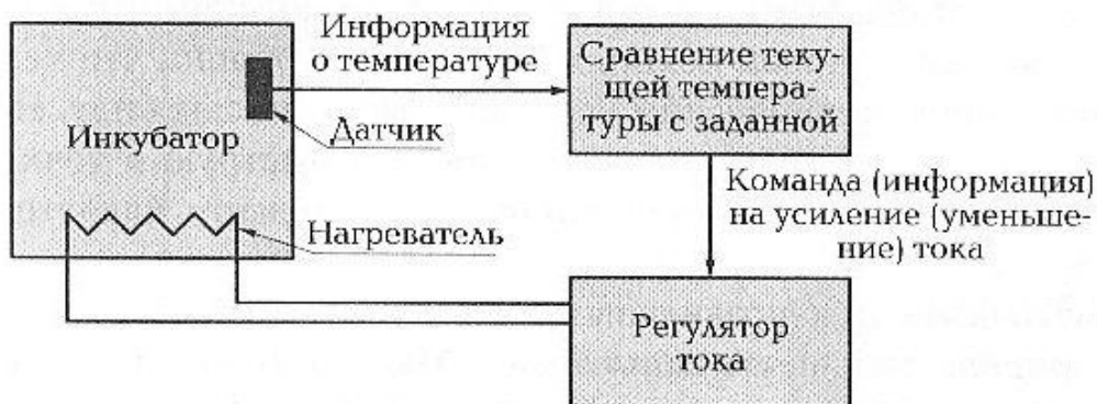
Рис. 2.3. Схема термостата
