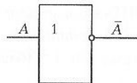
Рис. 3.10. Логическая схема НЕ
