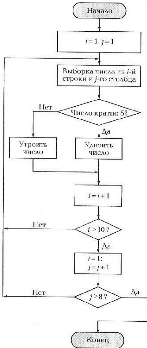
Рис. 2.36. Структурная схема алгоритма, использующего перебор элементов
