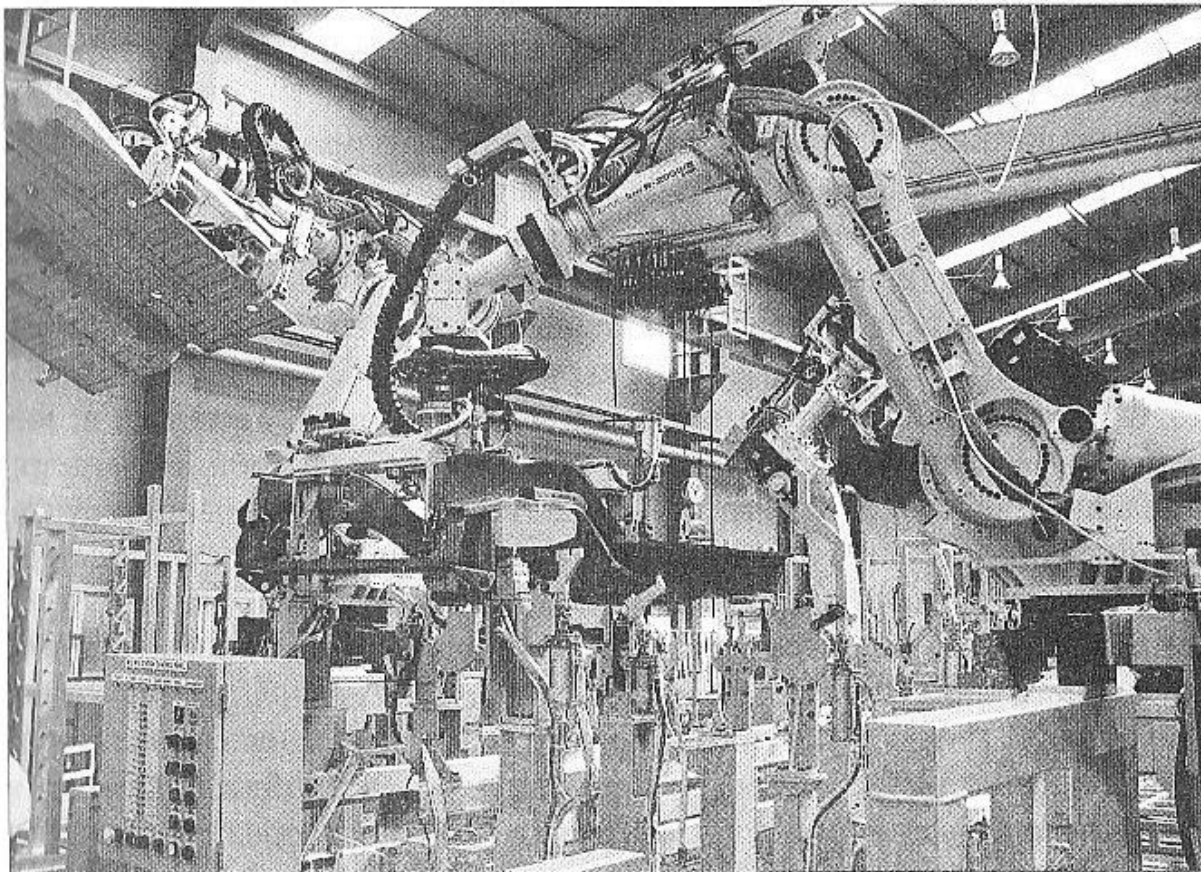
Рис. 1.3. Промышленный робот
